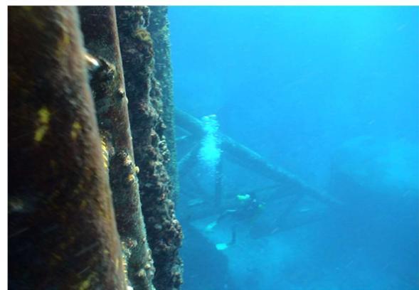
Khảo sát công trình Nhà giàn DK1 - Trường sa Surveying at DK1-Truong Sa construction
