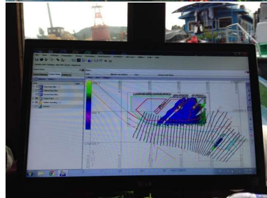
Khảo sát khu vực bến phao SPM và cảng xuất sản phẩm Jetty thuộc Nhà máy Lọc dầu Dung Quất/ Survey at Dung Quat refinery marine area
