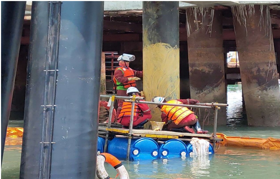
Thi công bọc cọc chống ăn mòn – Thanh Hóa Metal Anti-corrosion construction in Thanh Hoa
