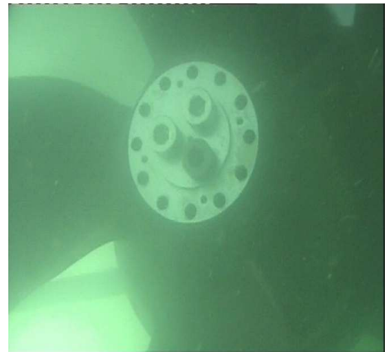
Khảo sát, quay phim chân vịt tàu SƠN DƯƠNG Making film underwater of SON DUONG vessel
